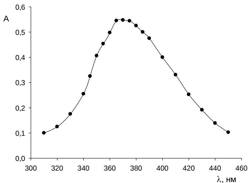
Рис. 4.12. Спектр поглощения при pH 2 нитрозо-Р-соли, иммобилизованной в желатиновой пленке (в растворе c(\text{HPC})=1.5 \cdot 10^{-3} моль/л).
