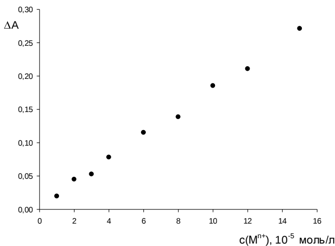
Рис. 5.7. Зависимость суммарного поглощения при pH 2 и \lambda=490 нм иммобилизованных в желатиновой пленке комплексов НРС с Co(II), Fe(III), Cu(II) и Ni(II) от суммарной концентрации ионов Co 2+ , Fe 3+ , Cu 2+ и Ni 2+ в растворе ( c(\sum M^{n+}) = \sum c(M^{n+}) , c(\text{Co}^{2+}) = c(\text{Cu}^{2+}) = c(\text{Ni}^{2+}) = c(\text{Fe}^{3+}) ).
