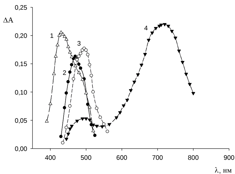
Рис. 4.13. Спектры поглощения при pH 2 комплексов ионов металлов с HPC, иммобилизованных в желатиновой пленке: 1 – Co(II), 2 – Ni(II), 3 – Cu(II), 4 – Fe(III) (в растворах: c(\text{Co}^{2+})=5 \cdot 10^{-5} моль/л, c(\text{Cu}^{2+})=c(\text{Ni}^{2+})=c(\text{Fe}^{3+})=1 \cdot 10^{-4} моль/л).
