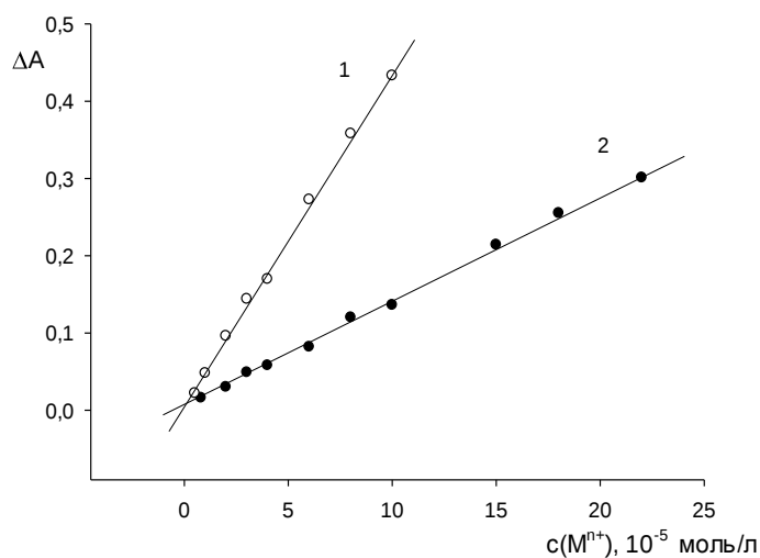
Рис. 5.5. Зависимость поглощения при рН 2 иммобилизованных в желатиновой пленке комплексов НРС с Co(II) (1) и Ni(II) (2) от концентрации ионов Co^{2+} и Ni^{2+} в растворе (1 – \lambda=430 нм, 2 – \lambda=470 нм).
