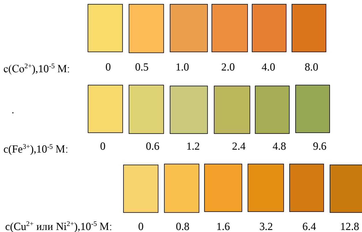
Рис. 5.4. Цветовые шкалы для тест-определения Co(II), Fe(III), Cu(II) и Ni(II) с использованием индикаторных НРС-пленок.
