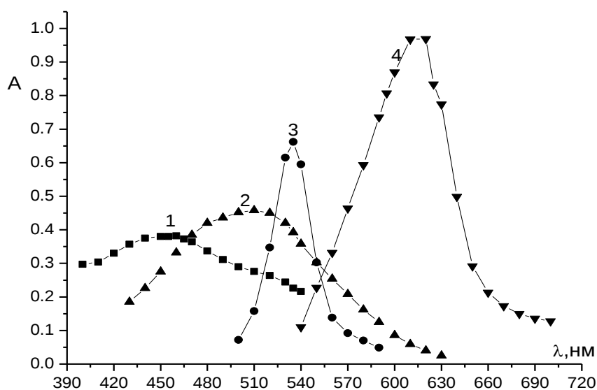
Рис. 4.18. Спектры поглощения иммобилизованных комплексов ионов \text{Al}^{3+} с АК (1) и ПКФ (2), иммобилизованных в желатиновой пленке (в растворах: 1 – c(\text{Al}^{3+})=2.0 \cdot 10^{-4} моль/л, pH 3.5; 2 – c(\text{Al}^{3+})=1.5 \cdot 10^{-4} моль/л, pH 6, c(\text{ЦПХ})=1.0 \cdot 10^{-4} моль/л).
