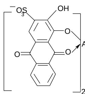
Al(АК)_2
