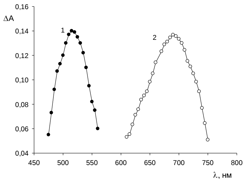
Рис. 4.18. Спектры поглощения иммобилизованных комплексов ионов \text{Al}^{3+} с АК (1) и ПКФ (2), иммобилизованных в желатиновой пленке (в растворах: 1 – c(\text{Al}^{3+})=2.0 \cdot 10^{-4} моль/л, pH 3.5; 2 – c(\text{Al}^{3+})=1.5 \cdot 10^{-4} моль/л, pH 6, c(\text{ЦПХ})=1.0 \cdot 10^{-4} моль/л).
