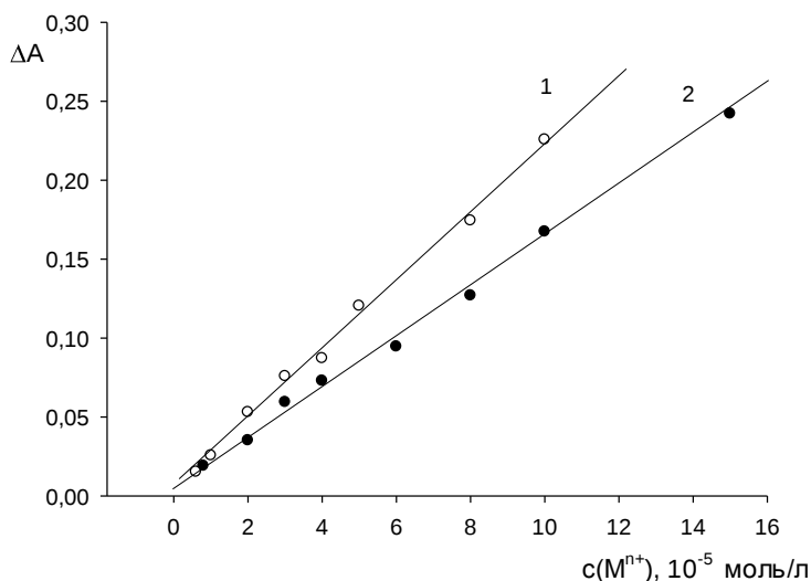
Рис. 5.6. Зависимость поглощения при pH 2 иммобилизованных в желатиновой пленке комплексов НРС с Fe(III) (1) и Cu(II) (2) от концентрации ионов Fe 3+ и Cu 2+ в растворе (1 – \lambda=720 нм, 2 – \lambda=495 нм).
