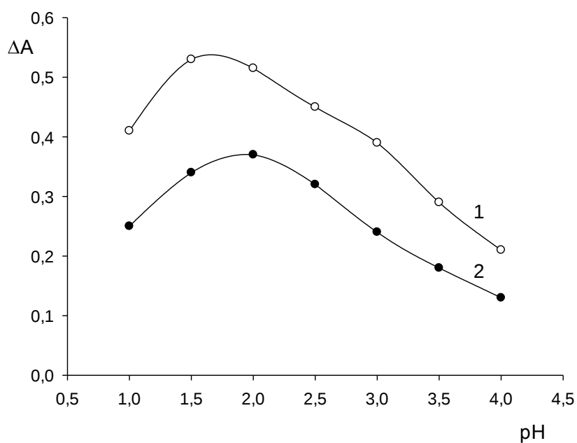
Рис. 4.6. Зависимость поглощения индикаторных пленок с иммобилизованными индикаторами нитхромазо (1) и АК (2) от кислотности растворов реагентов (1 — \lambda=590 нм, c(\text{нитхромазо})=3.0 \cdot 10^{-4} моль/л, t=20 мин; 2 — \lambda=435 нм, c(\text{АК})=5.0 \cdot 10^{-4} моль/л, t=20 мин).
