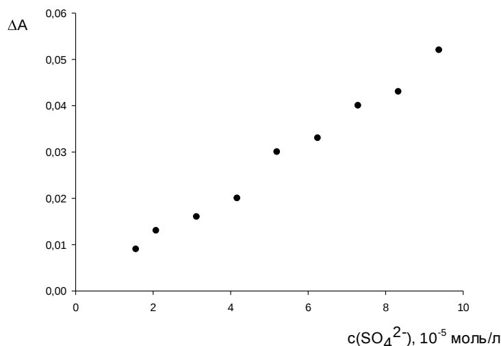
Рис. 5.9 Зависимость поглощения комплекса Ва(II) с нитхромазо в отвержденном желатиновом геле при \lambda = 675 нм от концентрации \text{SO}_4^{2-} в водно-этанольном растворе при pH 1.5.
