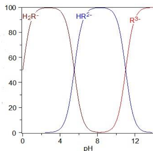
Рис. 4.3. Схемы протолитических равновесий (а, б) и долевая диаграмма распределения протонированных форм ализаринового красного S в зависимости от pH раствора ( K_{a2}=10^{-5.5} , K_{a3}=10^{-11.0} [203]).
