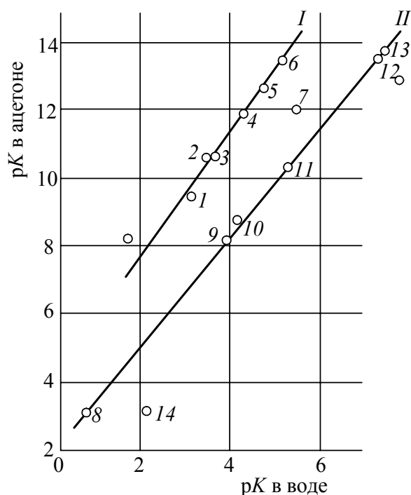
Рис. 2. Зависимость pK в ацетоне от pK в воде. I – ароматические карбоновые кислоты: 1 – салициловая, 2 – m -нитробензойная, 3 – n -нитробензойная, 4 – бензойная, 5 – n -оксибензойная, 6 – n -аминобензойная, 7 – антралиловая; II – фенолы: 8 – пикриновая кислота, 9 – 2,6-динитрофенол, 10 – 2,4-динитрофенол, 11 – 2,5-динитрофенол, 12 – n -нитрофенол, 13 – o -нитрофенол, 14 – сульфосалициловая кислота, 15 – сахарин [29].
