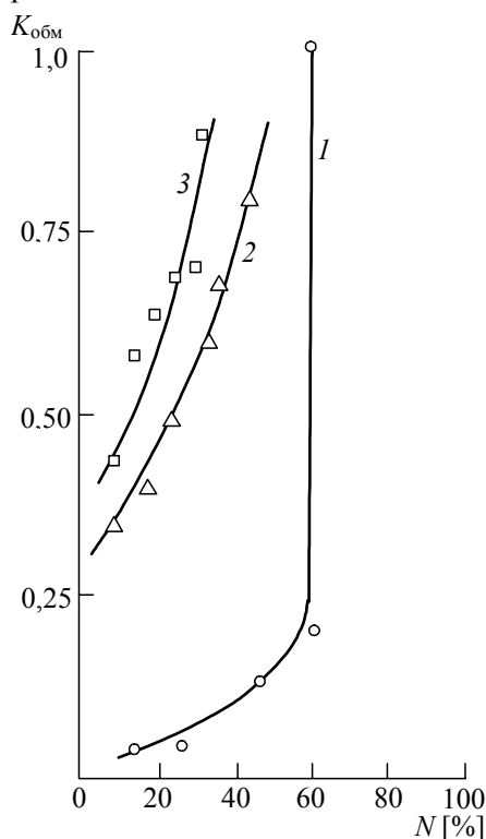
Рис. 1. Зависимость константы обмена ионов морфина на ион Ca^{2+} в воде и в смесях спирта с водой на катионите КУ-1 от степени использования емкости ионита органическим ионом. 1 – вода, 2 – 70%-ный этанол, 3 – 85%-ный этанол [28].
